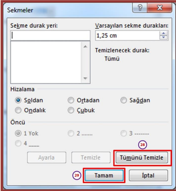
Şekil 5. Sekmeler Ayarları
